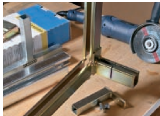
11. Sistemul de construcție modulară cu profile pentru susținerea unor instalații facilitează și realizarea unui perete cu rol de separare a spațiului.
